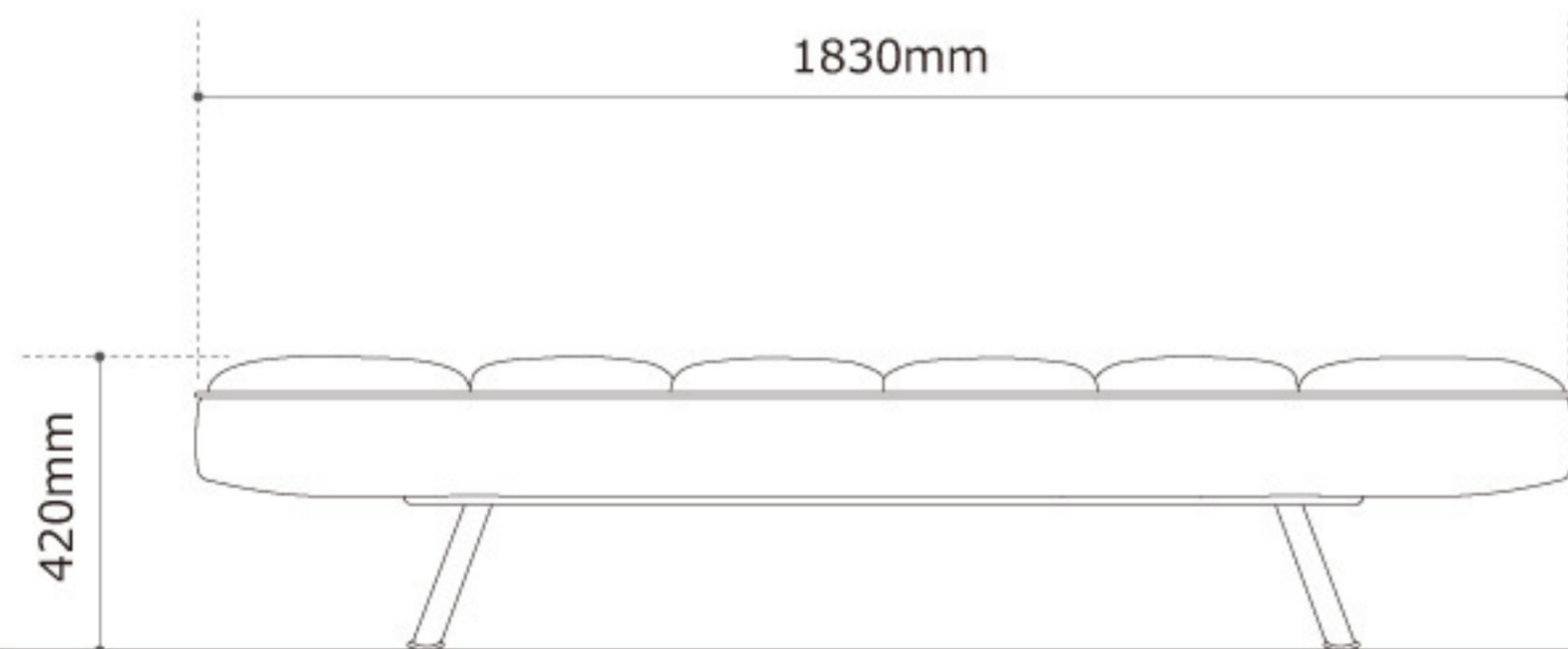
正面
