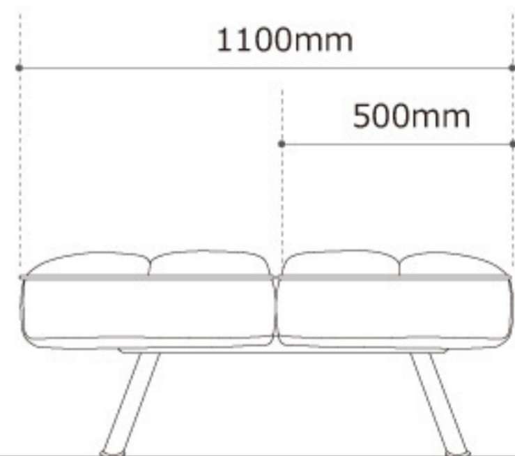
側面
